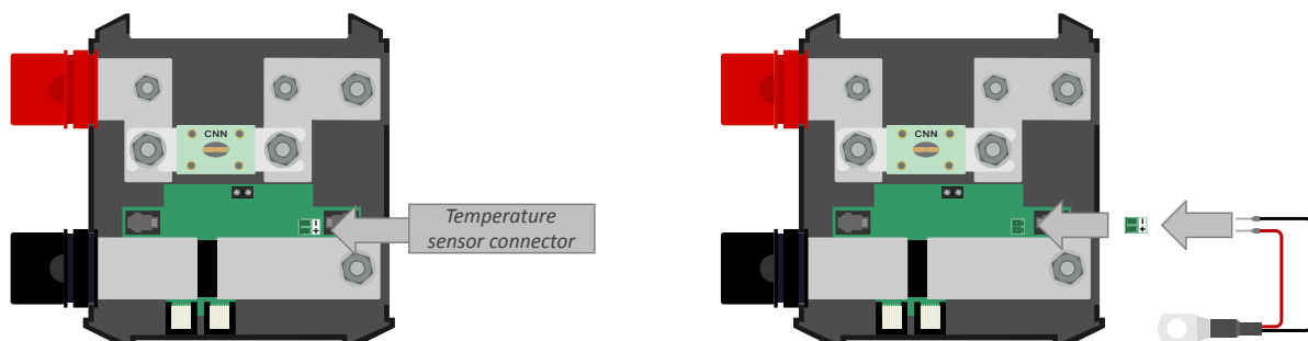
Temperatursensoranschluss Lynx Shunt VE.Can
